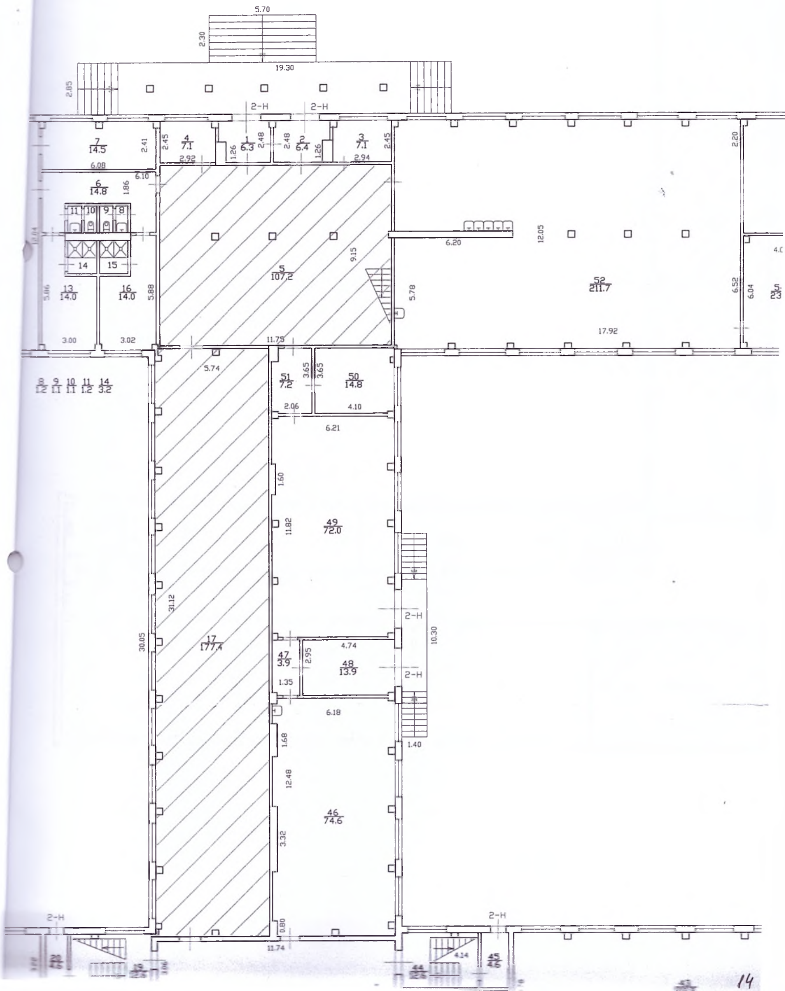
План 1 этажа
